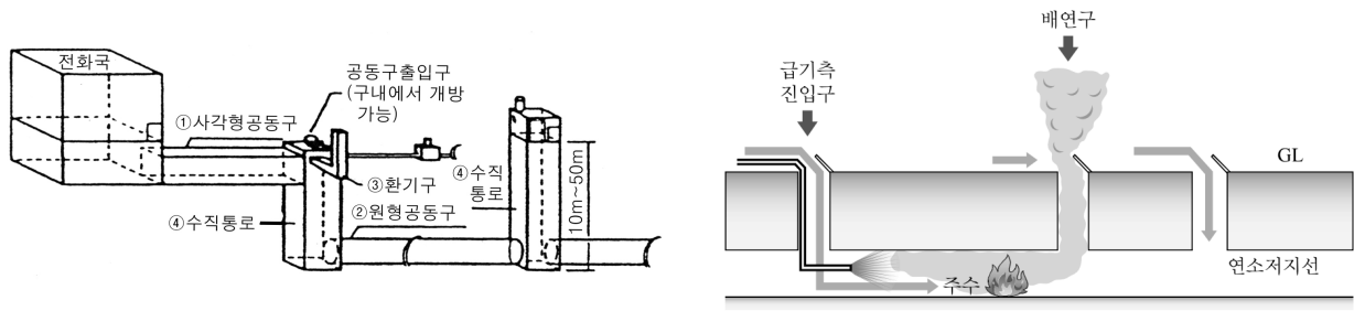
[그림 1-138] 공동구 계통도 / [그림 1-139] 공동구 화재 시 배연요령
